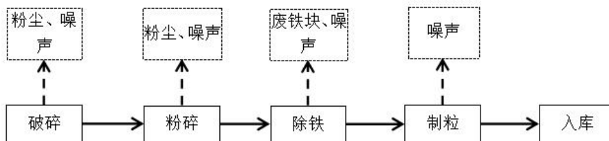
图 2 项目生产工艺流程图
