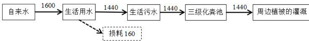
图 1 项目水平衡图（单位：m 3 /a）
